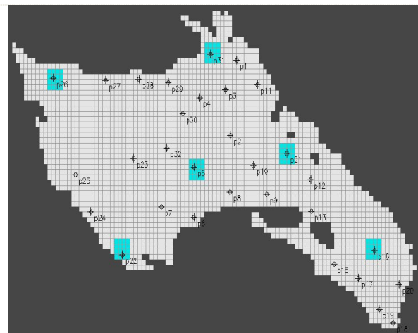
شکل ۵. موقعیت بلوک‌های انتخاب شده جهت انجام آنالیز حساسیت
