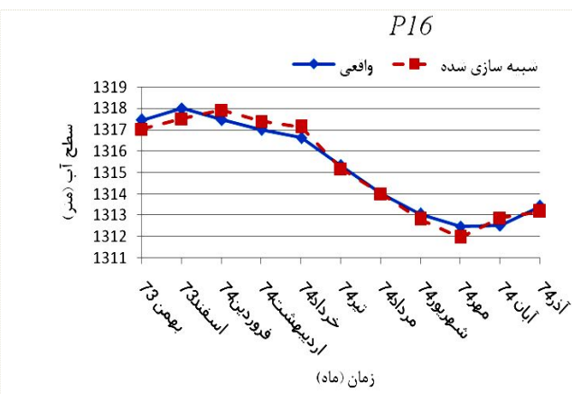
شکل ۷. نتایج واسنجی مدل در شرایط ناپایدار در دوره‌های زمانی پرپود ۶ و ۱۰
