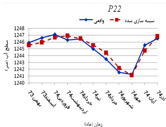
شکل ۷. نتایج واسنجی مدل در شرایط ناپایدار در دوره‌های زمانی پرپود ۶ و ۱۰
