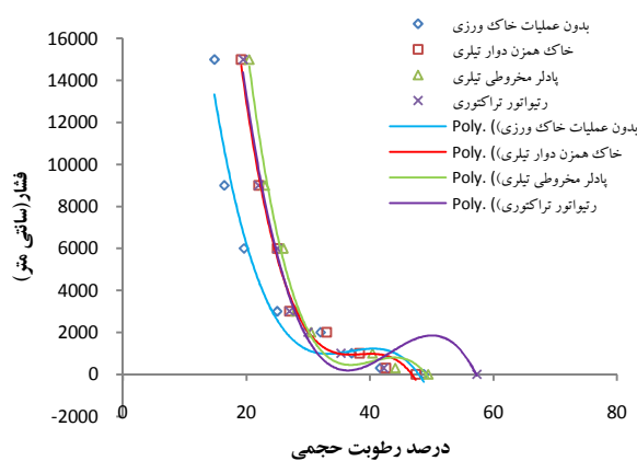
شکل ۱۱. مقایسه منحنی مشخصه خاک بدون عملیات خاک‌ورزی با خاک پادل شده با ادوات مختلف خاک‌ورزی
