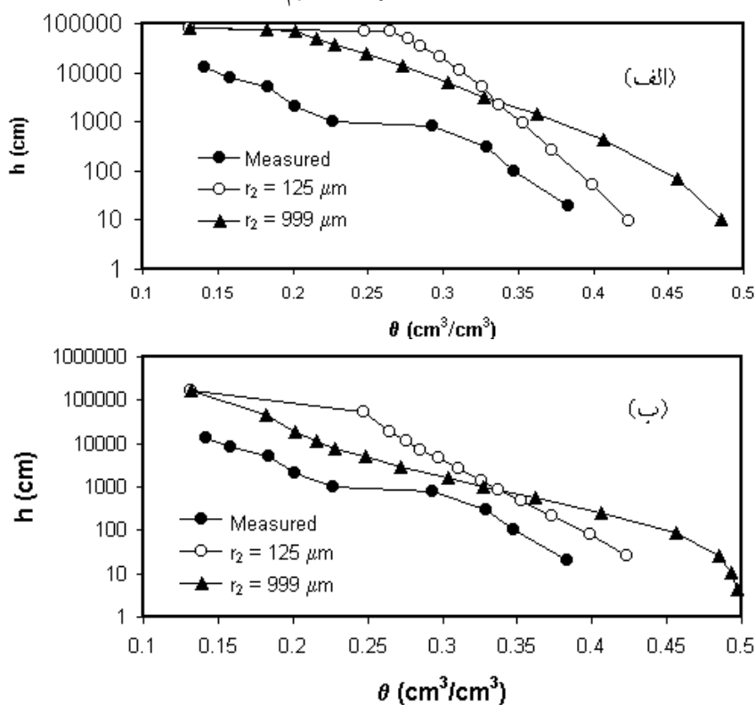
شکل ۶. منحنی مشخصه آب خاک بر مبنای \alpha محاسبه شده از روش لاجستیک (الف) و خطی (ب) و مقایسه با منحنی مشاهده‌ای در خاک ملاطانی (لوم)
