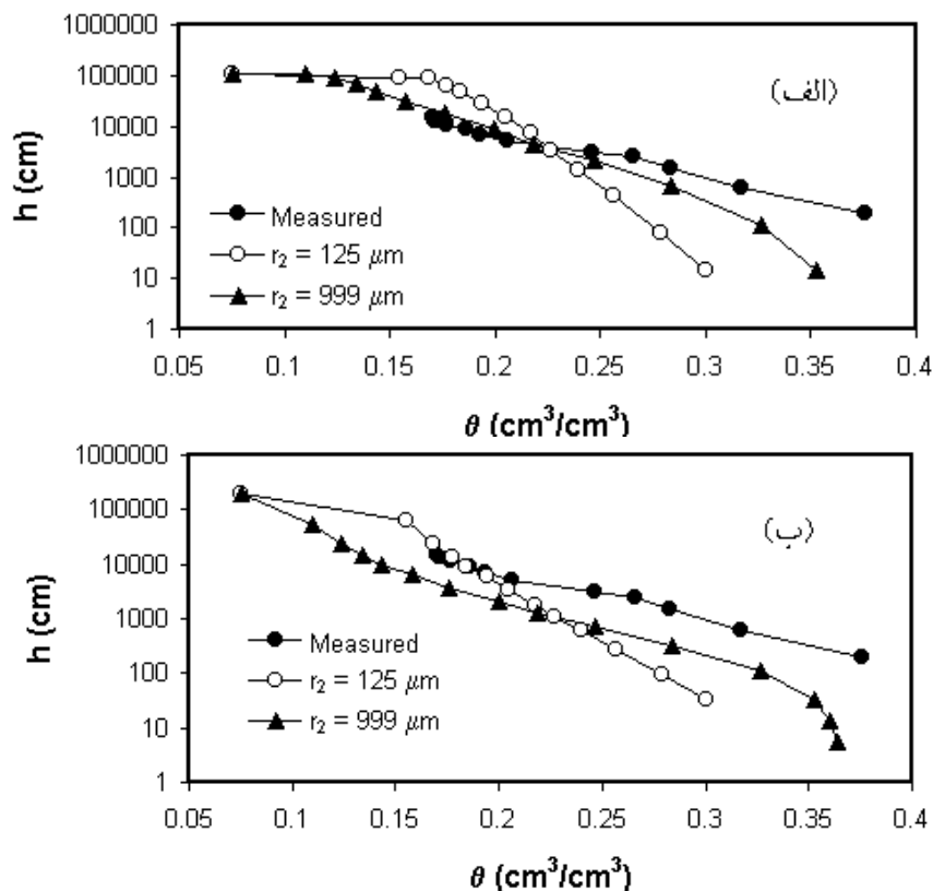
شکل ۵. منحنی مشخصه آب خاک بر مبنای \alpha محاسبه شده از روش لاجستیک (الف) و خطی (ب) و مقایسه با منحنی مشاهده‌ای در خاک سروستان (لوم)
