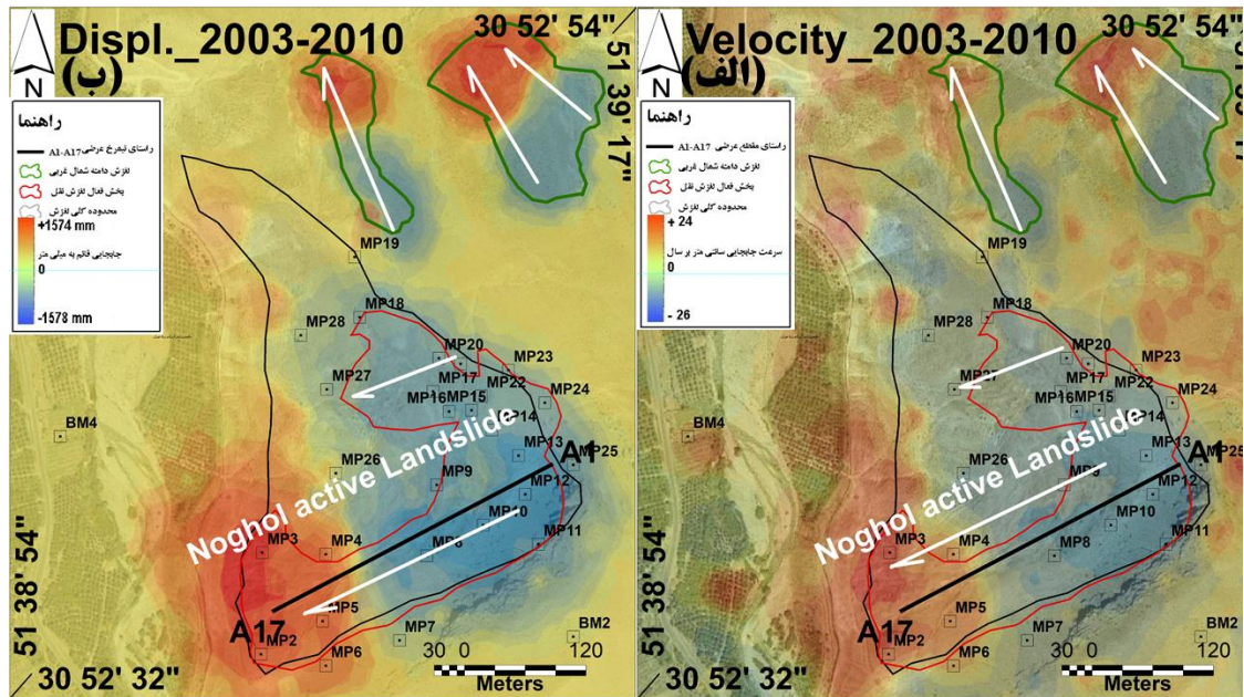
شکل ۱۰. نرخ جابه‌جایی زمین لغزش نقل در منطقه برداشت (مناطق آبی رنگ) و انباشتگی (مناطق قرمز رنگ) و نمایش نیمرخ طولی A1-A17 خط قرمز. محدوده لغزش فعال که با خط قرمز نشان داده شده است با توجه به برداشت های زمینی و تصاویر گوگل ارث ترسیم شده است (رنگی در نسخه الکترونیکی).
