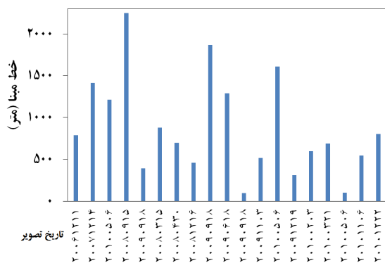
شکل ۵. توزیع مقادیر خط مبنای داده‌های ENVISAT ASAR (حرکت مداری: گذرپایین، گذر: ۳۳۵، زاویه فرود: ~ ۲۳°، سمت دید: راست، قطبش: HH)
