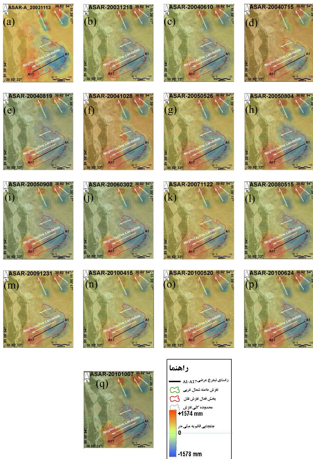
شکل ۸. نقشه‌های درون‌یابی حاصل از نقاط PS استخراج شده از تصاویر ASAR. طیف رنگ آبی نشانگر میزان جابه‌جایی در منطقه برداشت و طیف رنگ قرمز نماینده میزان جابه‌جایی در منطقه انباشتگی (رنگی در نسخه الکترونیکی)
