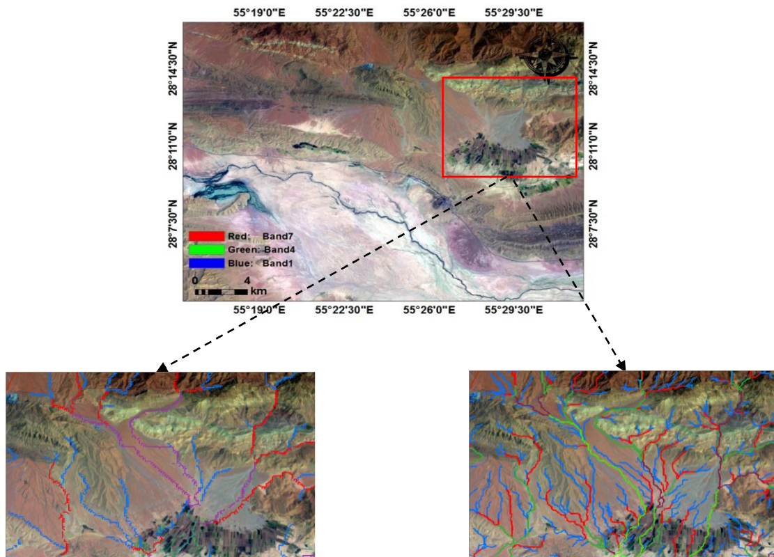
شکل ۸. موقعیت آبراهه‌ها بر روی تصاویر ماهواره‌ای لندست هشت (۲۰۱۵)
