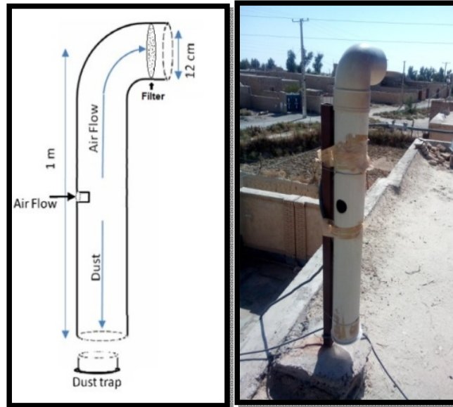
شکل ۲. نمونه رسوب‌گیر سیفونی مورد استفاده در تحقیق
