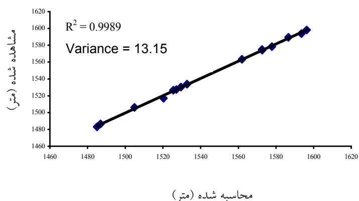
شکل ۴. مقادیر مشاهده شده نسبت به محاسبه شده برای گام زمانی ۱۲ از دوره تحریک ۴ در محل چاه‌های مشاهده‌ای
