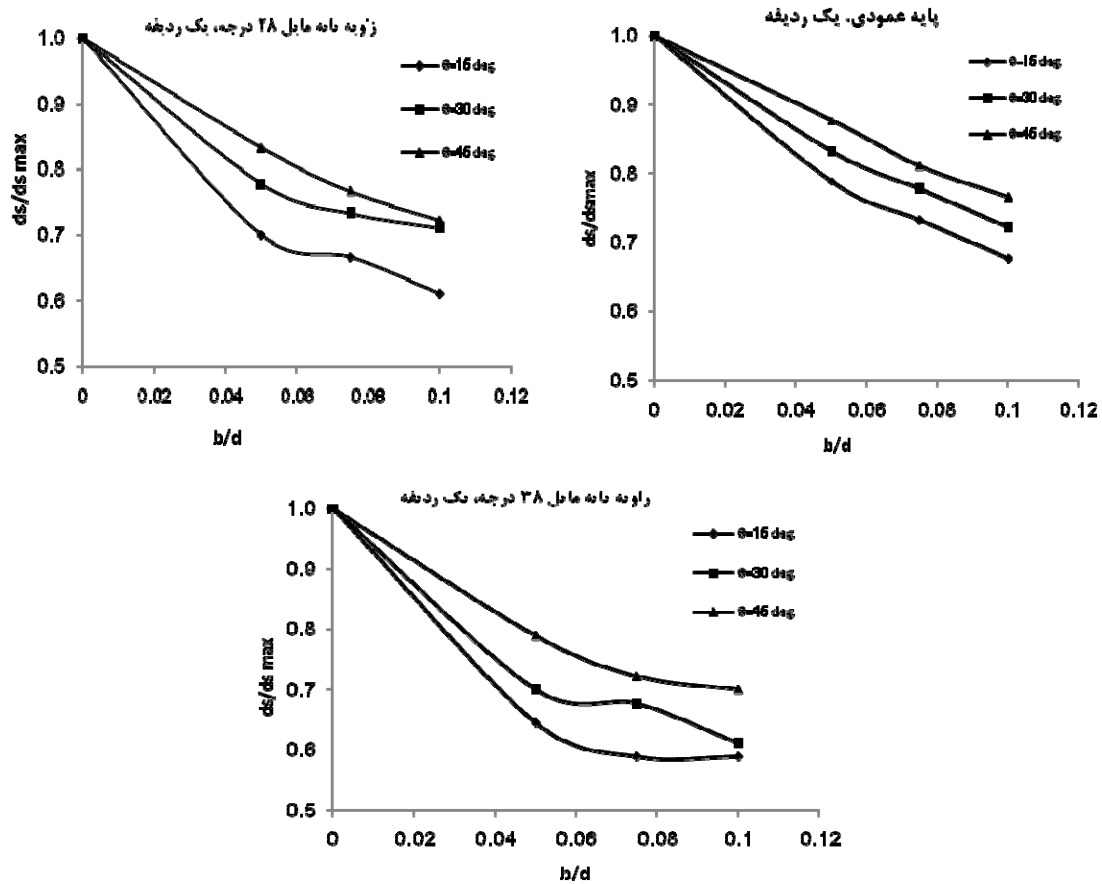
شکل ۶. تأثیر قطر نسبی کابل بر عمق آبشستگی در زاویه مختلف کابل و در سه زاویه پیش کابل و به صورت یک ردیفه
