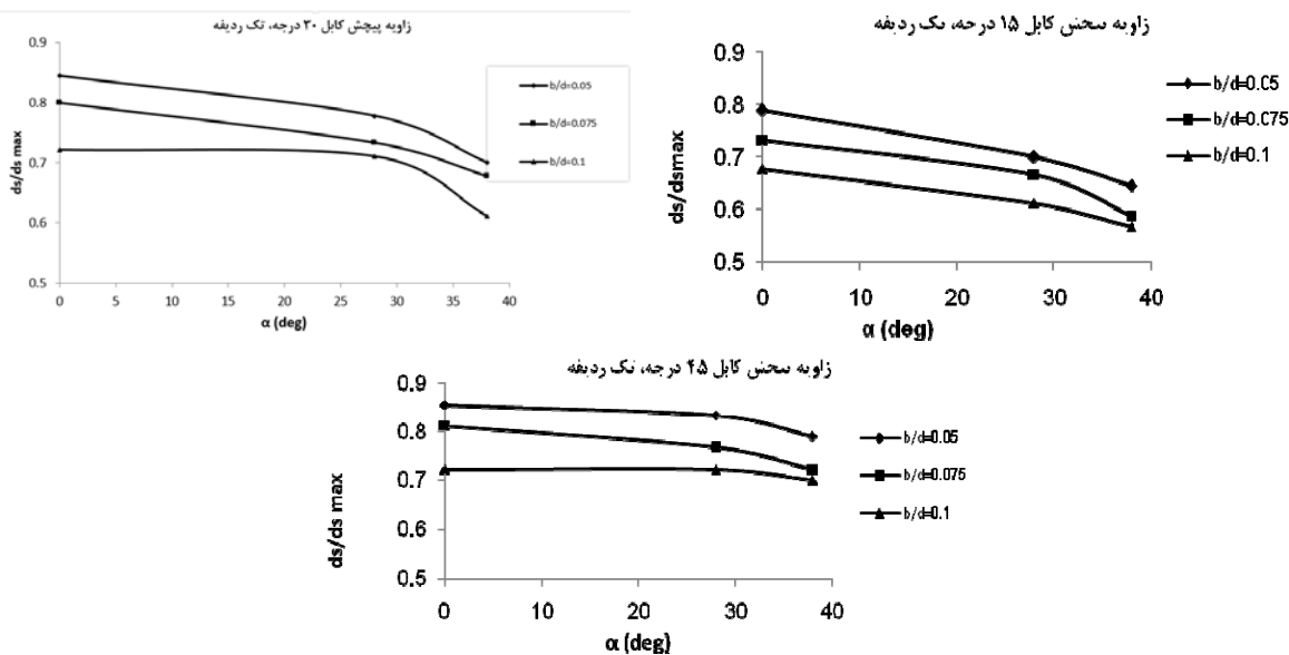
شکل ۸ تأثیر زاویه انحراف گروه پایه‌ها بر عمق آبستگي در سه قطر نسبي کابل و سه زاويه پيچش کابل برای شرایط یک ردیفه
