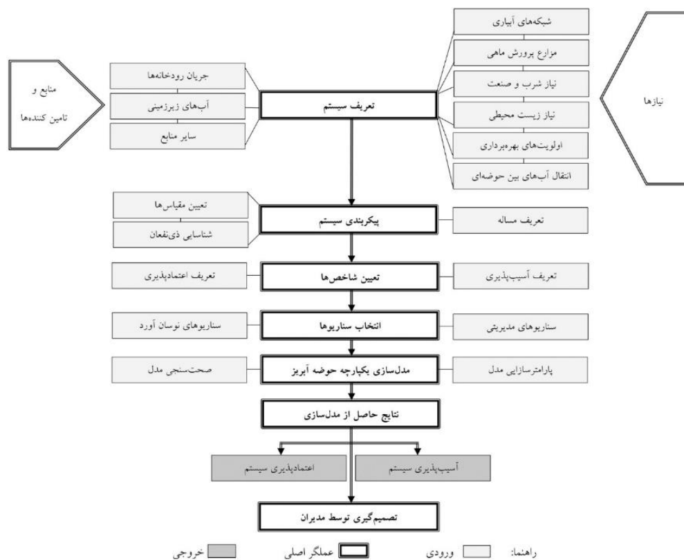
شکل ۵. مراحل شبیه‌سازی
