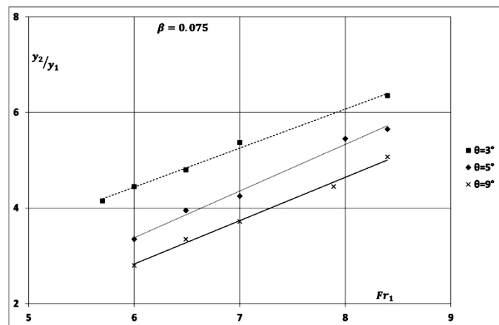
شکل ۱۱. تأثیر زاویه واگرایی بر عمق ثانویه نسبی در شیب کف ۷/۵ درصد و با وجود بلوک
