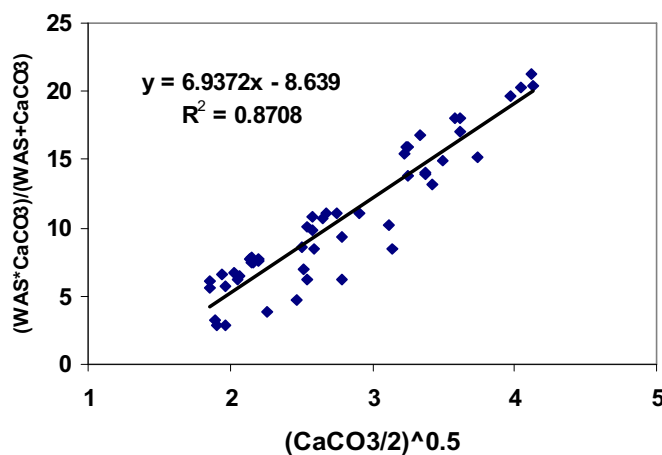
شکل ۷. نمودار رگرسیون خطی (پس از تبدیل متغیرها) یک متغیره رابطه WAS با آهک (CaCO 3 )
