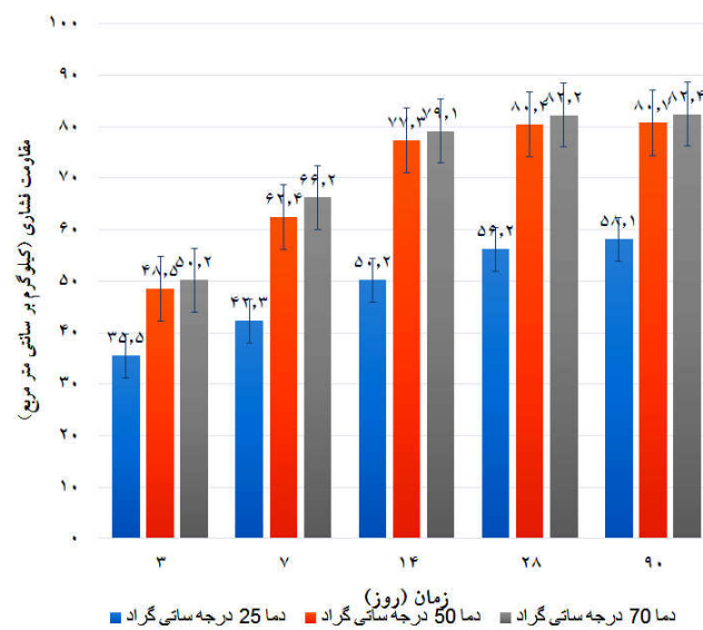
شکل ۷. تأثیر دما و زمان بر مقاومت باربری ژئوپلیمریزاسیون (رنگی در نسخه الکترونیکی)
