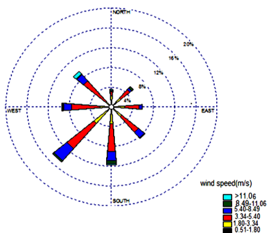
شکل ۲. گلباد متوسط سالانه شهرستان سیرجان
