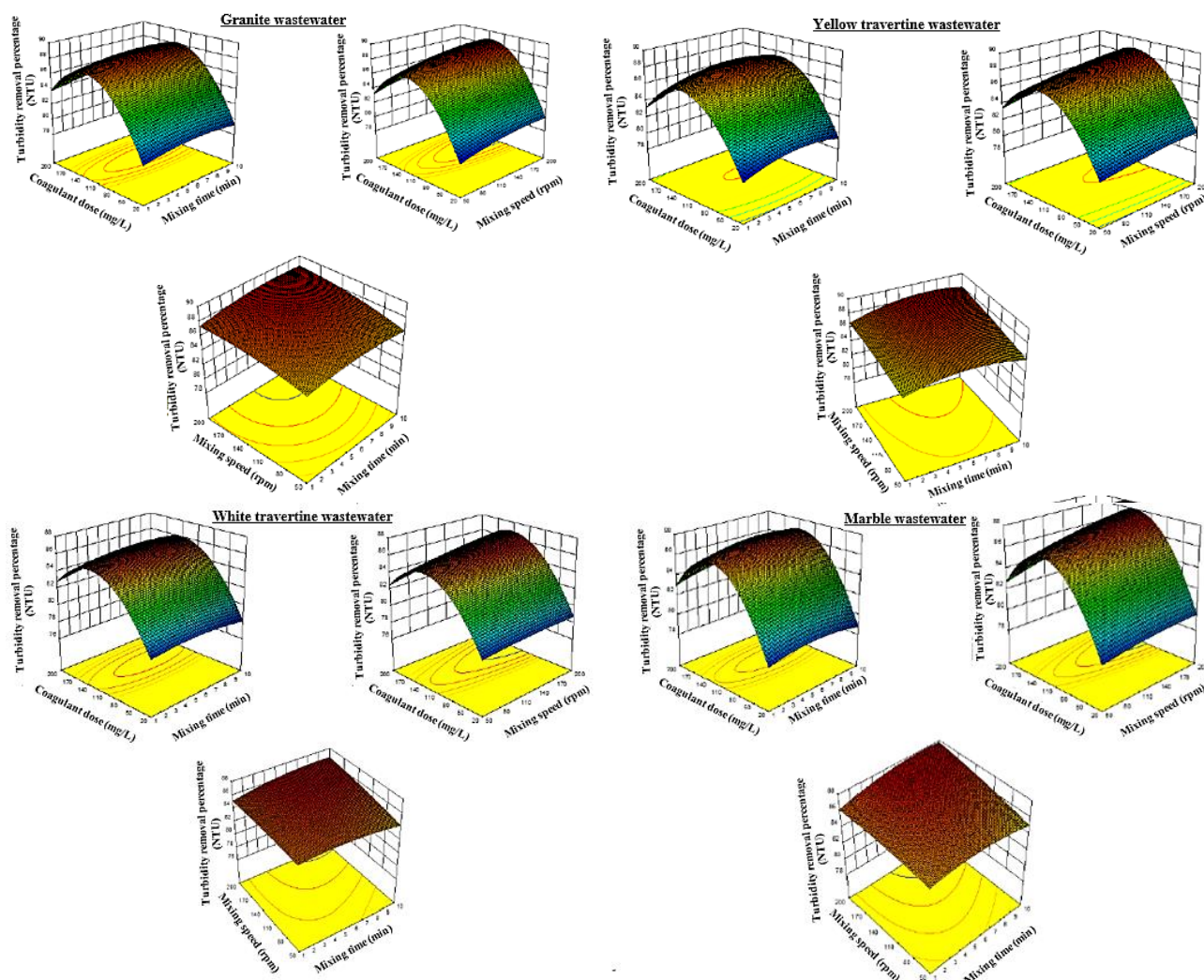
شکل ۴. اثر متقابل زمان اختلاط – دوز منعقدکننده، سرعت اختلاط – دوز منعقدکننده و زمان و سرعت اختلاط در حذف کدورت از ۴ نوع پساب سنگ‌بری با استفاده از سولفات آلومینیوم
