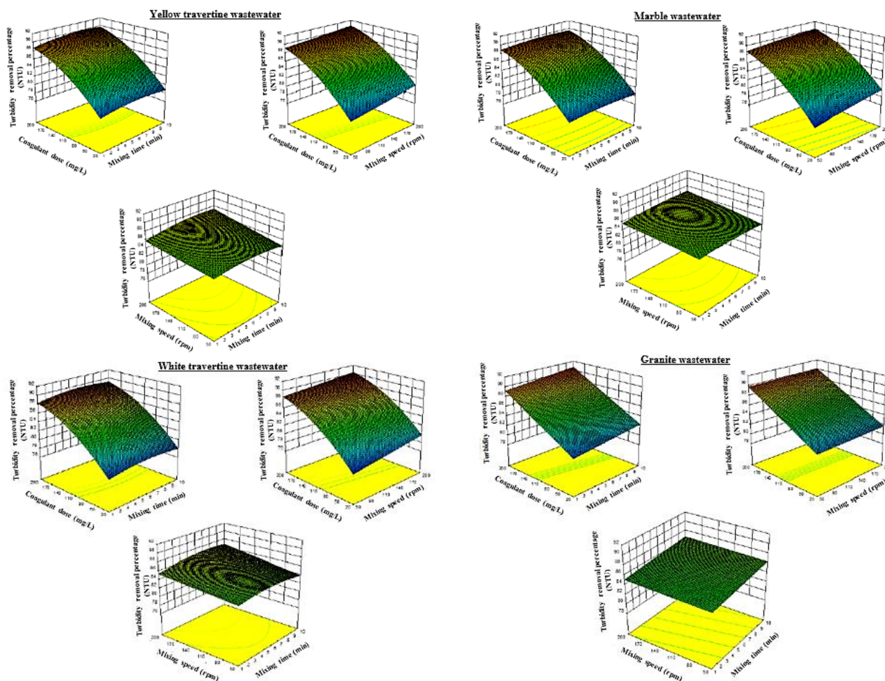
شکل ۳. اثر متقابل زمان اختلاط – دوز منعقدکننده، سرعت اختلاط – دوز منعقدکننده و زمان و سرعت اختلاط در حذف کدورت از ۴ نوع پساب سنگبری با استفاده از کلرید آهن
