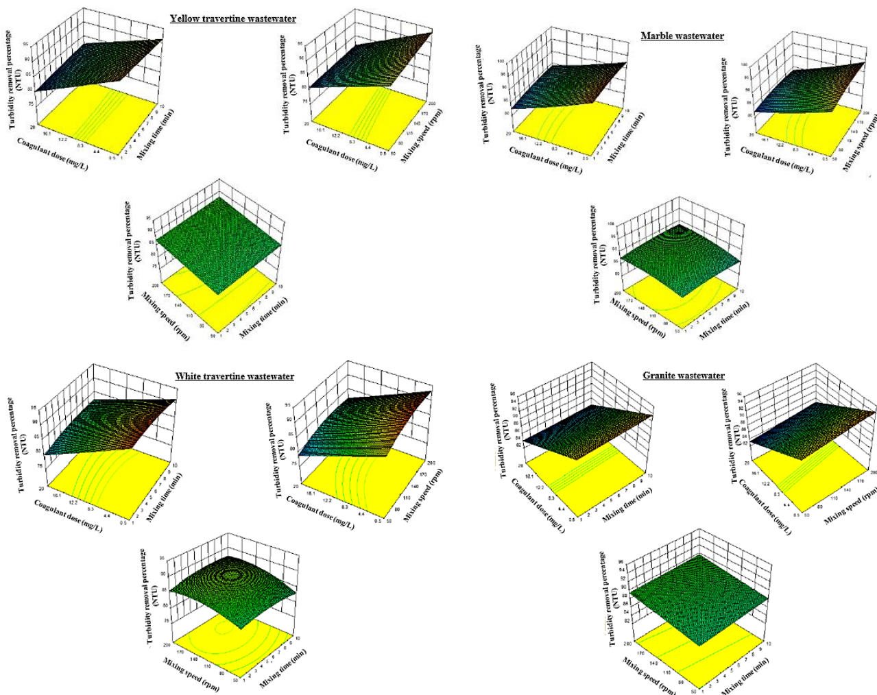
شکل ۵. اثر متقابل زمان اختلاط - دوز منعقدکننده، سرعت اختلاط - دوز منعقدکننده و زمان و سرعت اختلاط در حذف کدورت از ۴ نوع پساب سنگ‌بری با استفاده از پلی‌اکریل‌آمید کاتیونی
