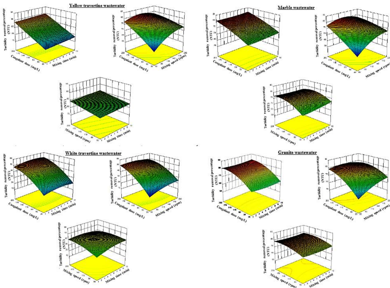
شکل ۱. اثر متقابل زمان اختلاط - دوز منعقدکننده، سرعت اختلاط - دوز منعقدکننده و زمان و سرعت اختلاط در حذف کدورت از ۴ نوع پساب سنگ‌بری با استفاده از زئولیت
