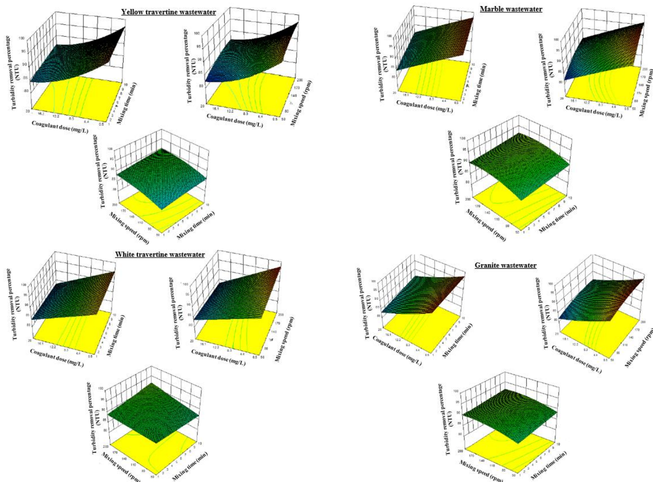
شکل ۶. اثر متقابل زمان اختلاط - دوز منعقدکننده، سرعت اختلاط - دوز منعقدکننده و زمان و سرعت اختلاط در حذف کدورت از ۴ نوع پساب سنگ‌بری با استفاده از پلی‌اکریل‌آمید آنیونی
