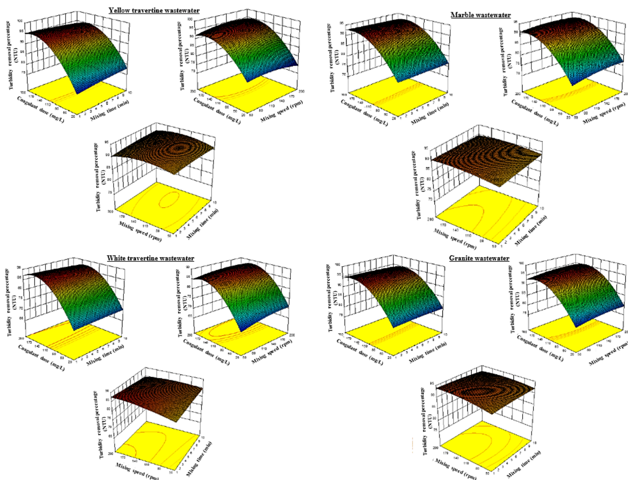
شکل ۲. اثر متقابل زمان اختلاط - دوز منعقدکننده، سرعت اختلاط - دوز منعقدکننده و زمان و سرعت اختلاط در حذف کدورت از ۴ نوع پساب سنگ‌بری با استفاده از پلی‌آلومینیوم کلراید
