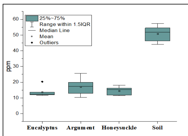
۳. محدوده غلظت سنجش شده نیکل (میلی گرم بر کیلوگرم) در نمونه های برگ اوکالپتوس، برهان، کهور و خاک کلانشهر اهواز Figure 3. Concentration range of nickel ( \text{mg kg}^{-1} ) in Eucalyptus globulus , Albizia lebbeck and Prosopis cineraria leaf samples and soil of Ahvaz metropolis
