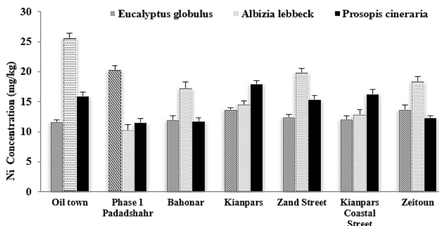
شکل ۱. مقایسه غلظت نیکل (میلی گرم بر کیلوگرم) برگ شسته شده درختان اوکالپتوس، برهان و کهور کلانشهر اهواز
