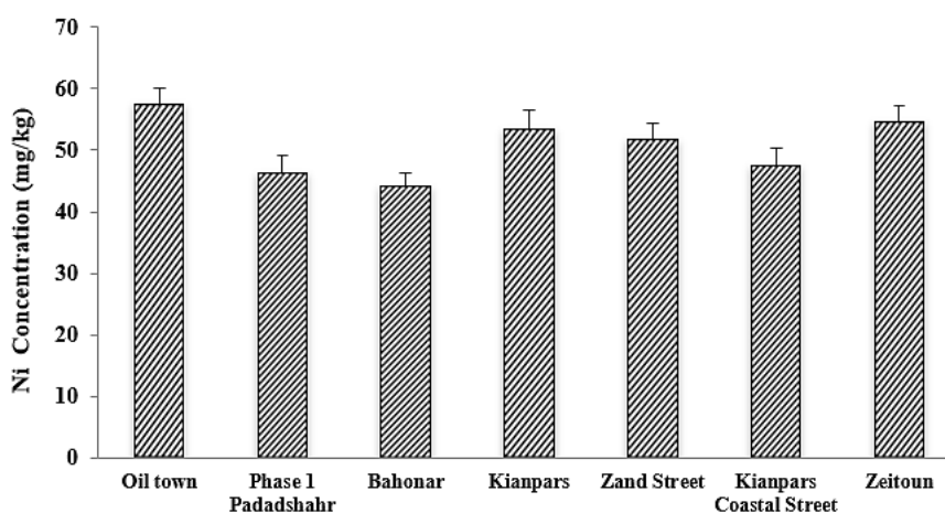
شکل ۴. مقایسه غلظت نیکل (میلی گرم بر کیلوگرم) در نمونه های خاک پای درختان مورد مطالعه کلانشهر اهواز Figure 4. Comparison of nickel concentration ( \text{mg kg}^{-1} ) in soil samples at the foot of trees studied in the Ahvaz metropolis
