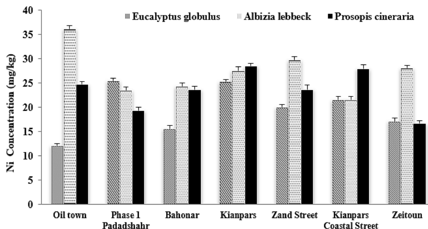
شکل ۲. مقایسه غلظت نیکل (میلی گرم بر کیلوگرم) برگ شسته نشده درختان اوکالپتوس، برهان و کهور کلانشهر اهواز Figure 2. Comparison of nickel concentration ( \text{mg kg}^{-1} ) of unwashed leaves of Eucalyptus globulus , Albizia lebbeck and Prosopis cineraria in Ahvaz metropolis
