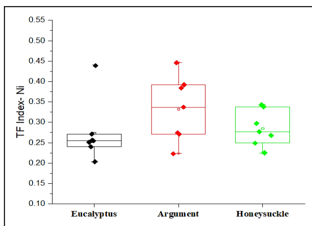
شکل ۶. مقایسه مقادیر شاخص فاکتور انتقال برای فلز سنگین نیکل در برگ گونه‌های اوکالپتوس، برهان و کهور
