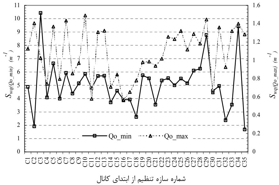
شکل ۵. مقادیر شاخص‌های حساسیت تغییرات نسبی بده به میزان بازشدگی سازه‌های تنظیم وادودارا در بده‌های بهره‌برداری مورد مطالعه
