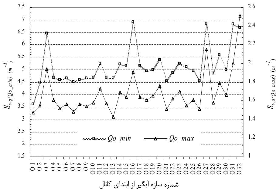
شکل ۶. مقادیر شاخص‌های حساسیت تغییرات نسبی بده به میزان بازشدگی سازه‌های آبگیر کانال وادودارا در بده‌های بهره‌برداری مورد مطالعه
