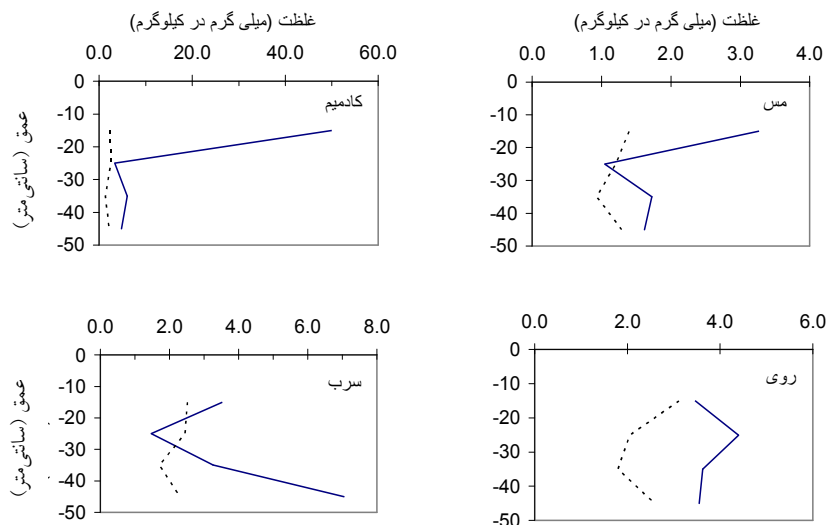
شکل ۴. مقایسه غلظت قابل عصاره‌گیری فلزات سنگین با DTPA در اعماق خاک در تیمارهای مختلف با اعداد نرمال شده غلظت‌های فلزات در تیمار آلوده تقسیم بر تیمار غیر آلوده مربوطه). تیمارها در صفحه ۵۸ توضیح داده شده‌اند. منحنی‌های خط شکسته مربوط به تیمارهای بدون کشت و خط کامل مربوط به تیمارهای کشت شده هستند.
