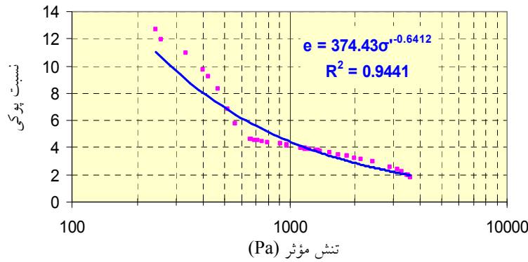
شکل ۸. رابطه بین تنش مؤثر و نسبت پوکي در آزمایش TA
