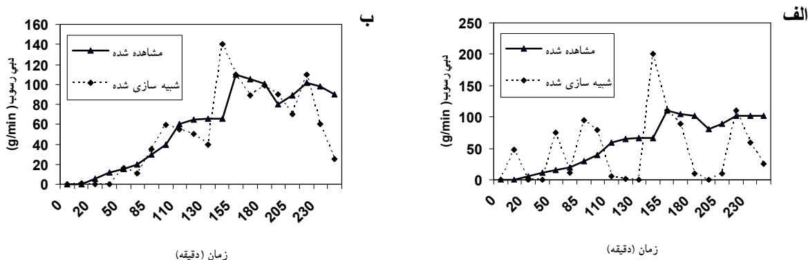
شکل ۵. منحنی واسنجی رسوب- زمان برای رخداد ۲۶ فروردین ۱۳۸۲ قبل (الف) و بعد (ب) از واسنجی به وسیله مدل EUROSEM در حوضه سولیجان
