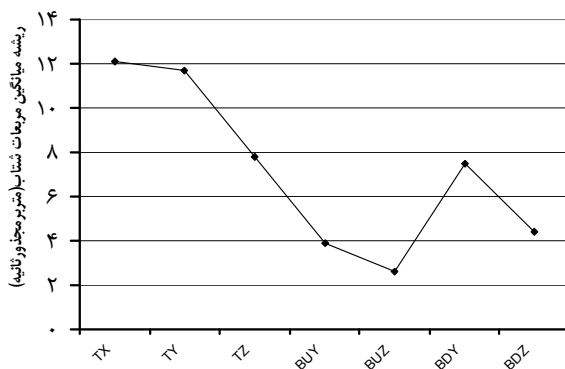
شکل ۱. مقادیر ریشه میانگین مربع‌های شتاب روی نیم تنه بالایی و نیم تنه پایینی بدن رانندگان و بدنه تراکتور را در راستاهای مختلف
