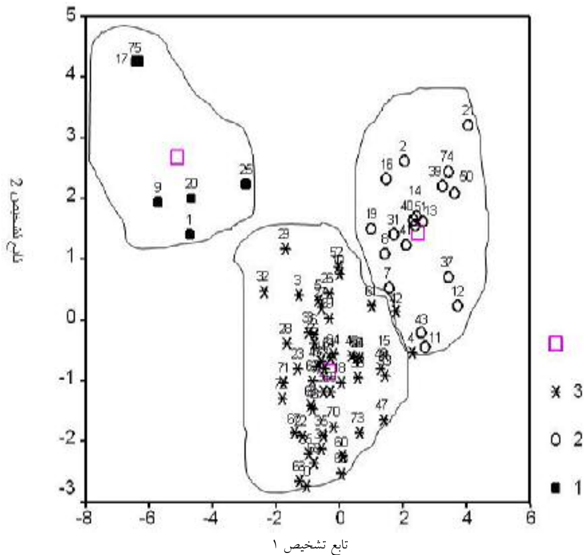
شکل ۲. نمودار تابع تشخیص در نقطه برش انتخاب شده در دندروگرام مربوط به شوری ۴ دسی زیمنس بر متر براساس صفات گیاهیچه‌ای. نام ژنوتیپ‌ها بر حسب شماره در شکل ۱ آمده است.
