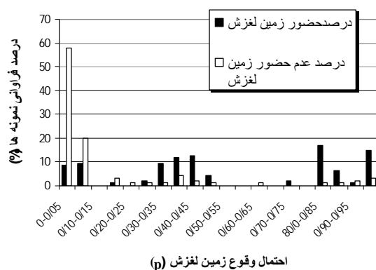
شکل ۳. درصد فراوانی حضور و عدم حضور لغزش در طبقات احتمال مختلف
