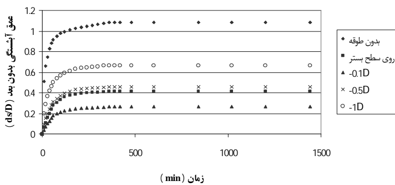
توسعه آبستگی با طوق W=2.5D
