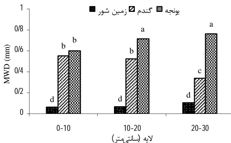
شکل ۳. مقایسه میانگین وزنی قطر خاک‌دانه‌ها (WMD) در لایه‌ها و کاربری‌های مختلف. مقایسه میانگین‌ها به روش LSD انجام شده و حروف مشابه در سطح ۰/۰۵ آماری بدون تفاوت معنی‌دار هستند (LSD = ۰/۰۸).
