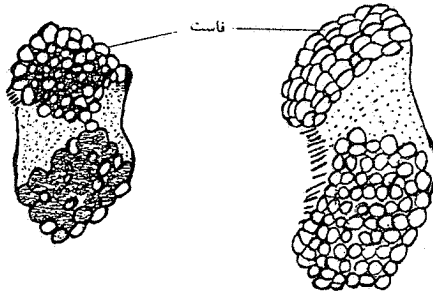
شکل ۲. چشم مرکب در T. vaporariorum (راست) و B. tabaci (چپ) (۴۰۰ برابر)
