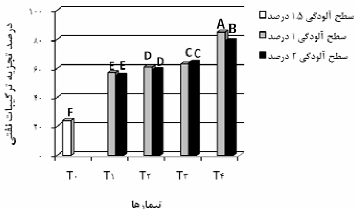
شکل ۱. راندمان تیمارهای T 0 : تیمار شاهد T 1 : تیمار کشت شبدر T 2 : کشت شبدر با مایه‌زنی میکوریزا T 3 : کشت شبدر با مایه‌زنی باکتری‌های تجزیه‌گر T 4 : کشت شبدر با مایه‌زنی میکوریزا و باکتری‌های تجزیه‌گر برای تجزیه هیدروکربن‌های نفتی در سطوح مختلف آلودگی
