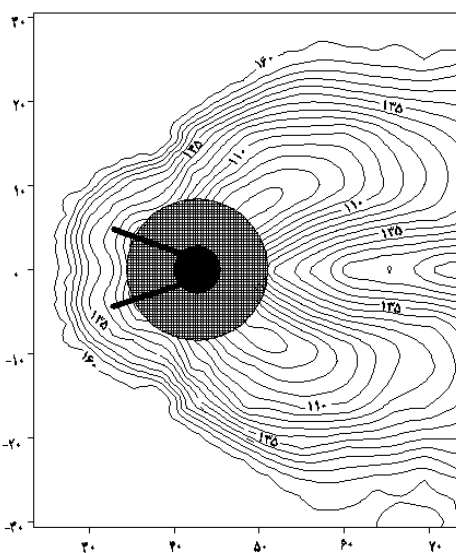
شکل ۷. خطوط میزان دو بعدی حفره آبستگی آزمایش G_1
