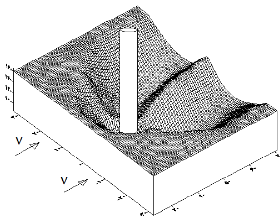
شکل ۶. توپوگرافی حفره آبستگی آزمایش G_1
