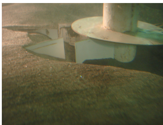
شکل ۸. حفره آبستگی پس از ۲۴ ساعت در آزمایش G_2
