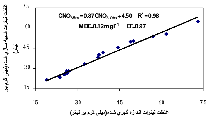
شکل ۷. روند تغییرهای غلظت نیترات اندازه گیری شده و شبیه سازی شده در آب زیرزمینی کرت مورد بررسی
