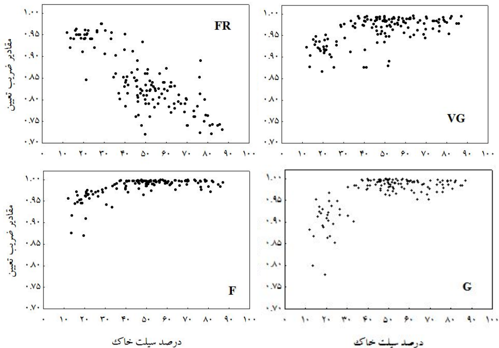
شکل ۹. رابطه بین ضرایب تعیین چهار مدل PSD ون گنوختن، فراکتال، گمپرتز و فردلانند با درصد سیلت نمونه‌های خاک. (VG = مدل ون گنوختن، FR = مدل فراکتال، G = مدل گمپرتز و F = مدل فردلانند)
