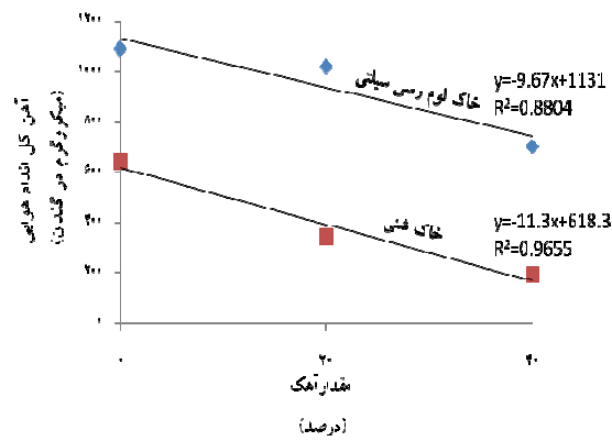
شکل ۲. اثر مقادیر مختلف کربنات کلسیم بر جذب آهن کل اندام هوایی توسط ذرت در دو نوع بافت خاک (هر نقطه میانگین ۹ داده است).
