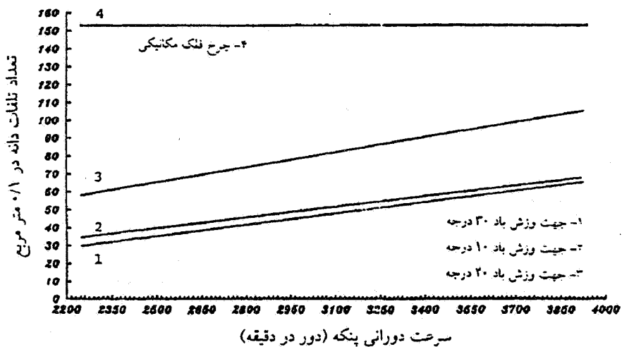
شکل ۱۳. تلفات دانه توسط چرخ فلک مکانیکی و بادی در ۱/۱ مترمربع، برحسب دور پنکه
