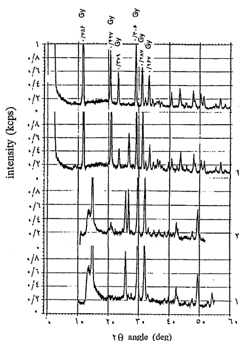
شکل ۳- منحنیهای پراش اشعه ایکس ذرات کمتر از ۰/۲ میلیمتر سازند شمشک ۱- گچ خالص با تیمار ۱۱۰°C حرارت ۲- ذغال سنگ رگه هیدروترومال با تیمار ۱۱۰°C ۳- پودر ذغال سنگ رگه هیدروترومال ۴- گچ خالص
