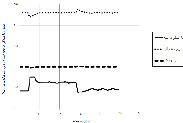
شکل ۸. تغییرات تراز سطح آب و دبی دریافتی در محل آبگیر شماره ۴ و بازشدگی سازه تنظیم کننده مربوط به آبگیر
