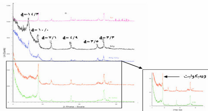
شکل ۹. الگوی پراش اشعه x کانی‌های مقطع کنترل رطوبتی خاک آلفی سولز
