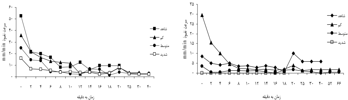
الف) سرعت نفوذ در شدت ترافیک‌های مختلف در مسیر چوبکشی ۱-۵ سال (ب) سرعت نفوذ در شدت ترافیک‌های مختلف در مسیر چوبکشی ۵-۱۰ سال
