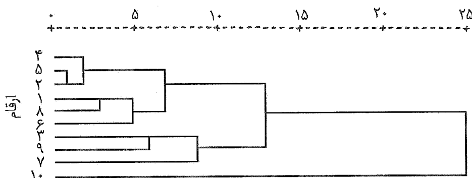
شکل ۱- دندروگرام ارقام سویای مورد مطالعه در خولنجان اصفهان. شماره‌های ۱ تا ۱۰ به ترتیب مربوط به ارقام ویلیامز، وودورث، هاک، زان، بلاک هاک، بونوس، استیل، اس.ار.اف، هارکور و هاییت می باشد.
