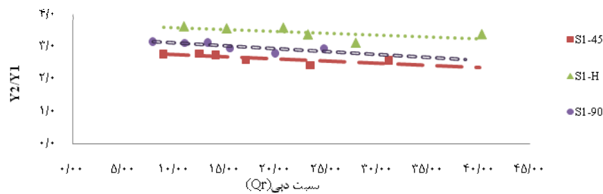
شکل ۹. تغییرات نسبت اعماق مزدوج پرش هیدرولیکی به نسبت دبی شکاف در مدل S ۱
