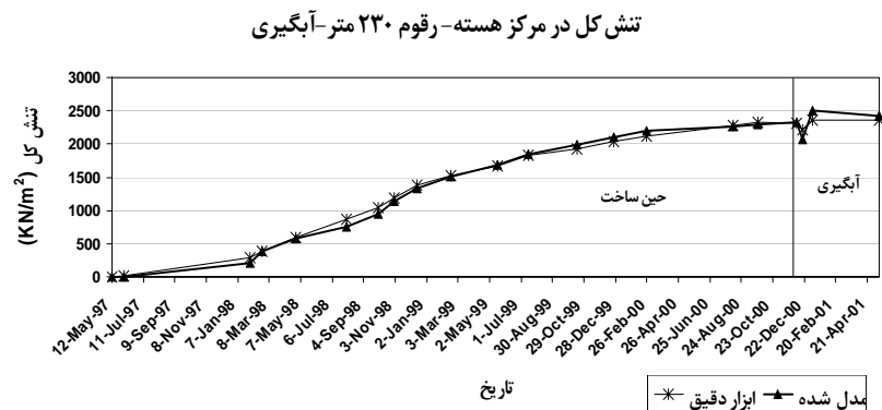
شکل ۹. نتایج فشار آب منفذی، نسبت فشار آب منفذی و تنش کل مدل شده و حاصل از ابزار دقیق در ابزار PPE212 و EP2103
