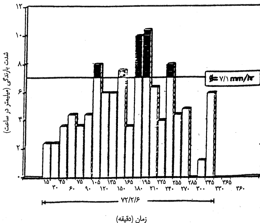
شکل ۳- هیئوگراف بارندگی در ایستگاه بوئین (مورخ ۶ اردیبهشت ۱۳۷۲)
