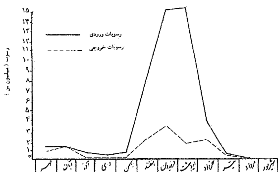
شکل ۲- تغییرات ورودی و خروجی رسوب سد سپیدرود در ماههای مختلف سال، قبل از عملیات شاس (۴)
