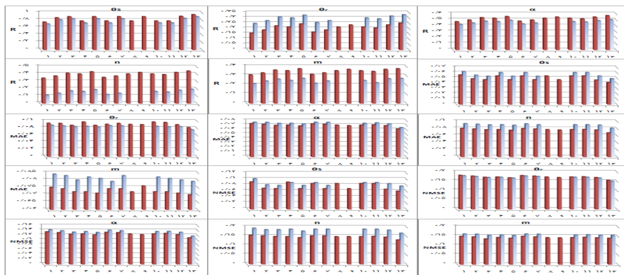
شکل ۴. مقادیر آماره‌های ارزیابی عملکرد برای ترکیب‌های مختلفی از متغیرهای ورودی (مدل‌های ۱ تا ۱۳) در برآورد پارامتریک معادله فردلند و زینگ به وسیله شبکه عصبی MLP برای دو عمق ۴۰- (رنگ قرمز) و ۸۰- سانتی متری (رنگ آبی)
