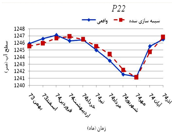
شکل ۷. نتایج واسنجی مدل در شرایط ناپایدار در دوره‌های زمانی پریود ۶ و ۱۰
