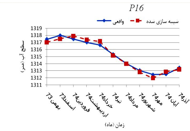
شکل ۷. نتایج واسنجی مدل در شرایط ناپایدار در دوره‌های زمانی پریود ۶ و ۱۰
