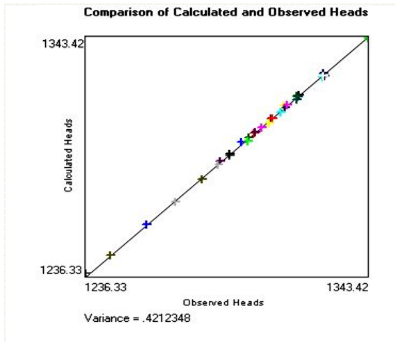
شکل ۶. نتیجه واسنجی مدل در شرایط پایدار
