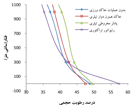
شکل ۱۲. مقایسه منحنی مشخصه خاک بدون عملیات خاک‌ورزی و خاک پادله شده با ادوات خاک‌ورزی مختلف در فشار اشباع، ظرفیت زراعی (۳۰۰ سانتی متر)، آستانه ترک بحرانی (۱۰۰۰ سانتی متر)
