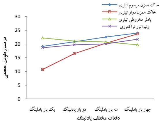
شکل ۷. مقایسه اثر ادوات خاک‌ورزی بر درصد رطوبت حجمی خاک در نقطه پژمردگی دائم
