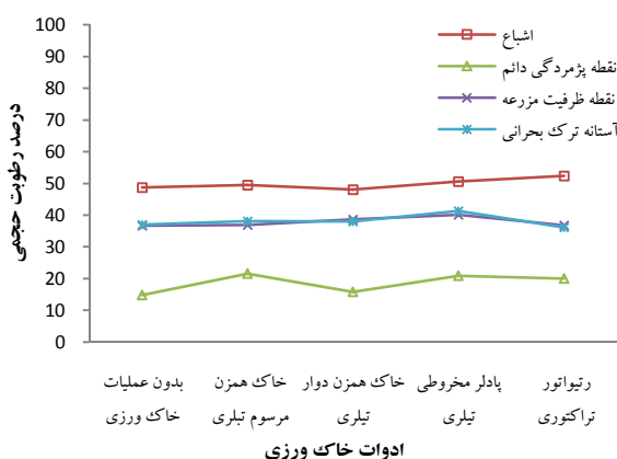
شکل ۵. مقایسه درصد رطوبت حجمی در نقطه اشباع و
