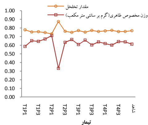
شکل ۱۴. مقایسه روند تخلخل و وزن مخصوص ظاهری برای ادوات مختلف خاک‌ورزی با دفعات مختلف پادلینگ
