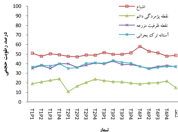
شکل ۴. روند تغییرات درصد رطوبت حجمی در نقطه اشباع و پژمردگی
