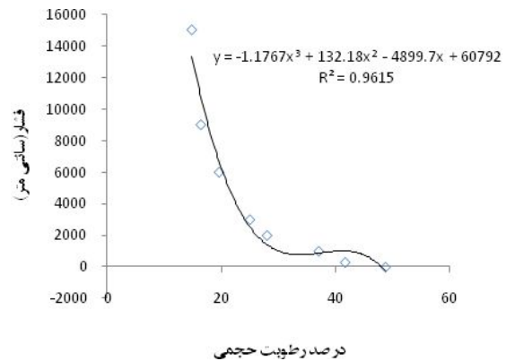
شکل ۱۰. منحنی مشخصه رطوبتی خاک بدون عملیات خاک ورزی
