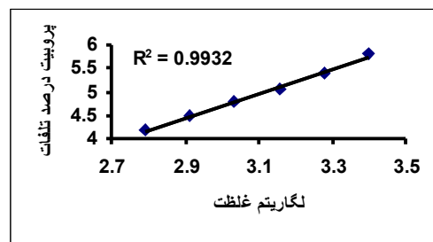
شکل ۳. رابطه بین لگاریتم غلظت و پروبیت درصد تلفات سن سوم
