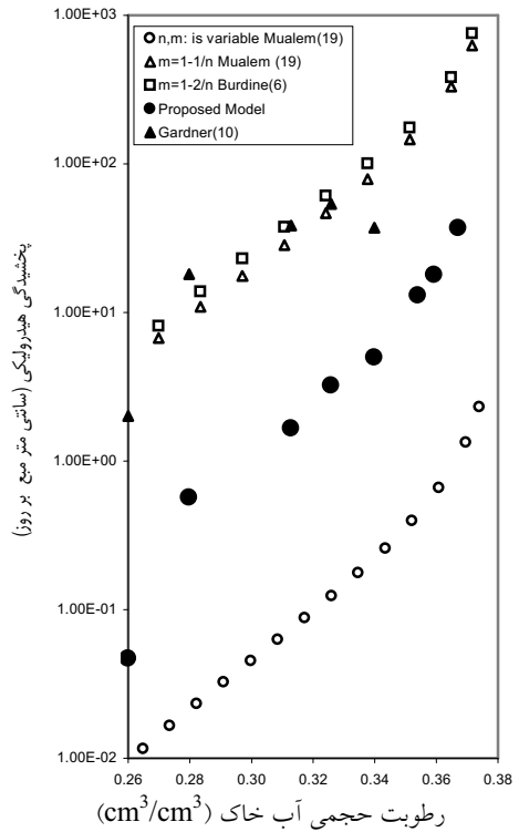
شکل ۱۵. پخشیدگی هیدرولیکی در خاک دیزج سیایش (بافت لومی رسی)
