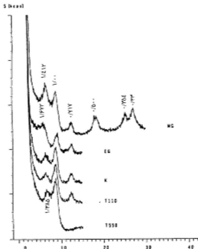
شکل ۵. پراش نگاشت‌های پرتو X ذرات رس ریز افق Bz نیم‌ریخ دشت دامنه‌ای (pp)
