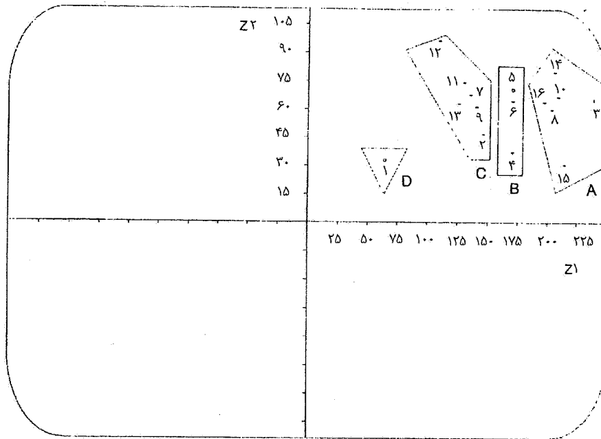
شکل ۴- نقشه پراکندگی ۱۶ توده بومی پیاز برووی دو مؤلفه اصلی Z_1 و Z_2 با استفاده از روش تجزیه به مؤلفه‌های اصلی
