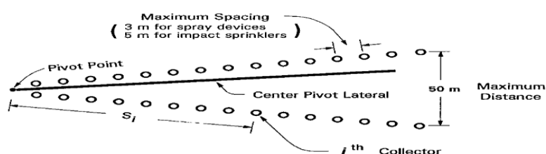
شکل ۳. نحوه چینش قوطی‌ها طبق استاندارد انجمن مهندسين کشاورزي آمريکا
