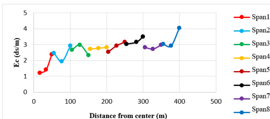
شکل ۹. نمودار شوری خاک در اسپن‌های مختلف دستگاه
