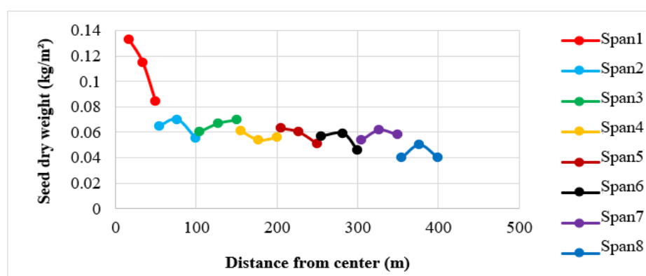
شکل ۶. وزن دانه کلزا در اسپن‌های مختلف دستگاه
