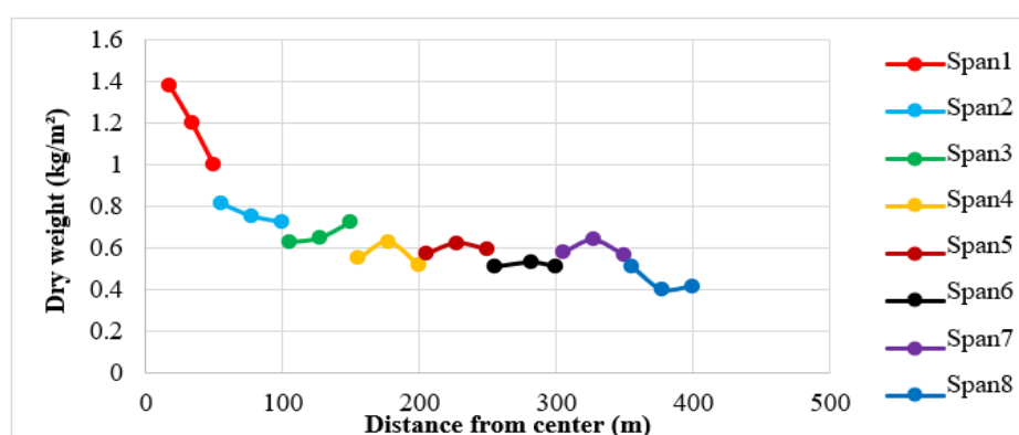
شکل ۵. وزن خشک کلزا در اسپن‌های مختلف دستگاه
