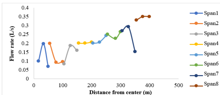
شکل ۷. دبی آبیاش‌ها در اسپن‌های مختلف دستگاه
