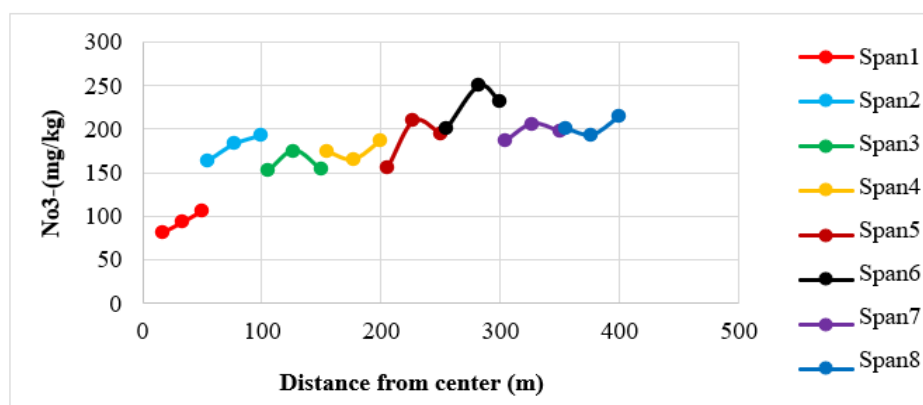
شکل ۸. نیترات باقیمانده در خاک در اسپن‌های مختلف دستگاه
