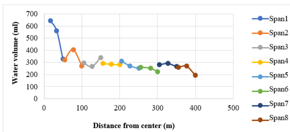
شکل ۴. میانگین حجم آب جمع شده در قوطی‌ها
