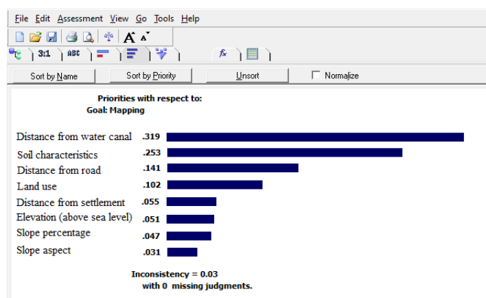
شکل ۲. نتایج حاصل از وزن‌دهی به معیارها و زیرمعیارها با استفاده از تحلیل سلسله مراتبی Figure 2. Results of weighting criteria and sub-criteria using Analytic Hierarchy Process
