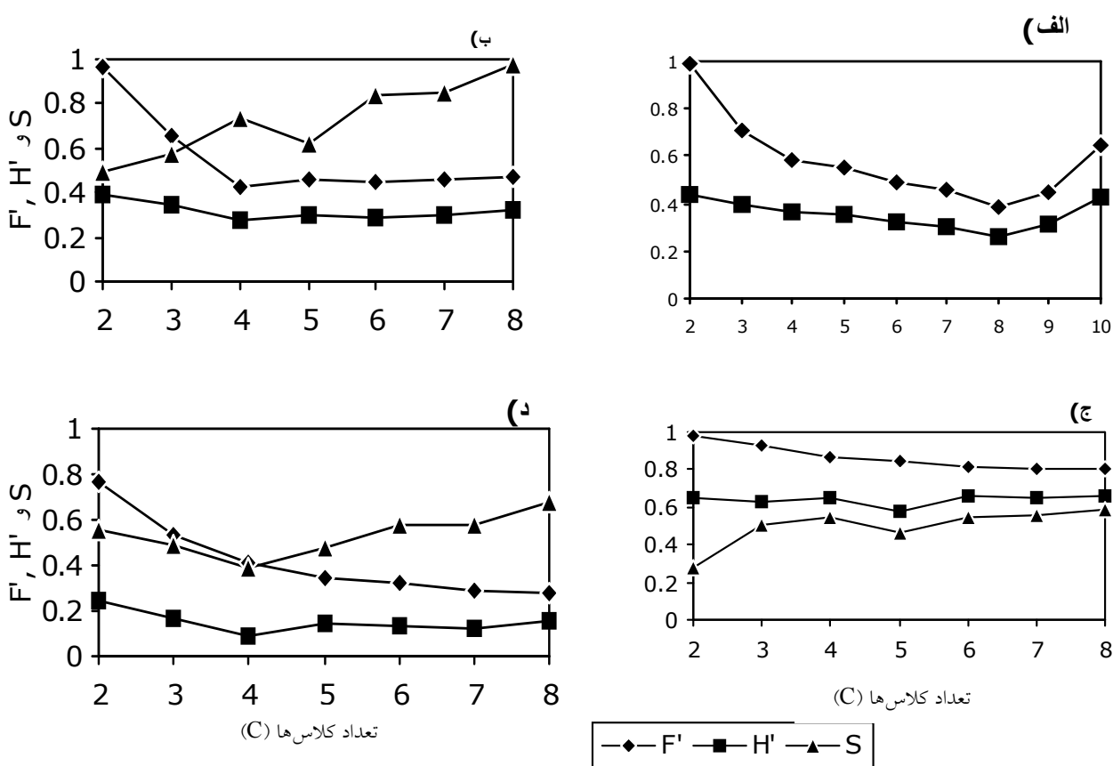
شکل ۲. تغییرات F' ، H' و S بر حسب تعداد کلاسها برای زیر مجموعه‌های: کل با نمای فازی ۱/۲۷ (الف)، ریخت شناختی با نمای فازی ۱/۴۵ (ب)، و بافت با نمای فازی ۱/۱۶ (ج) و ۱/۳ (د)
